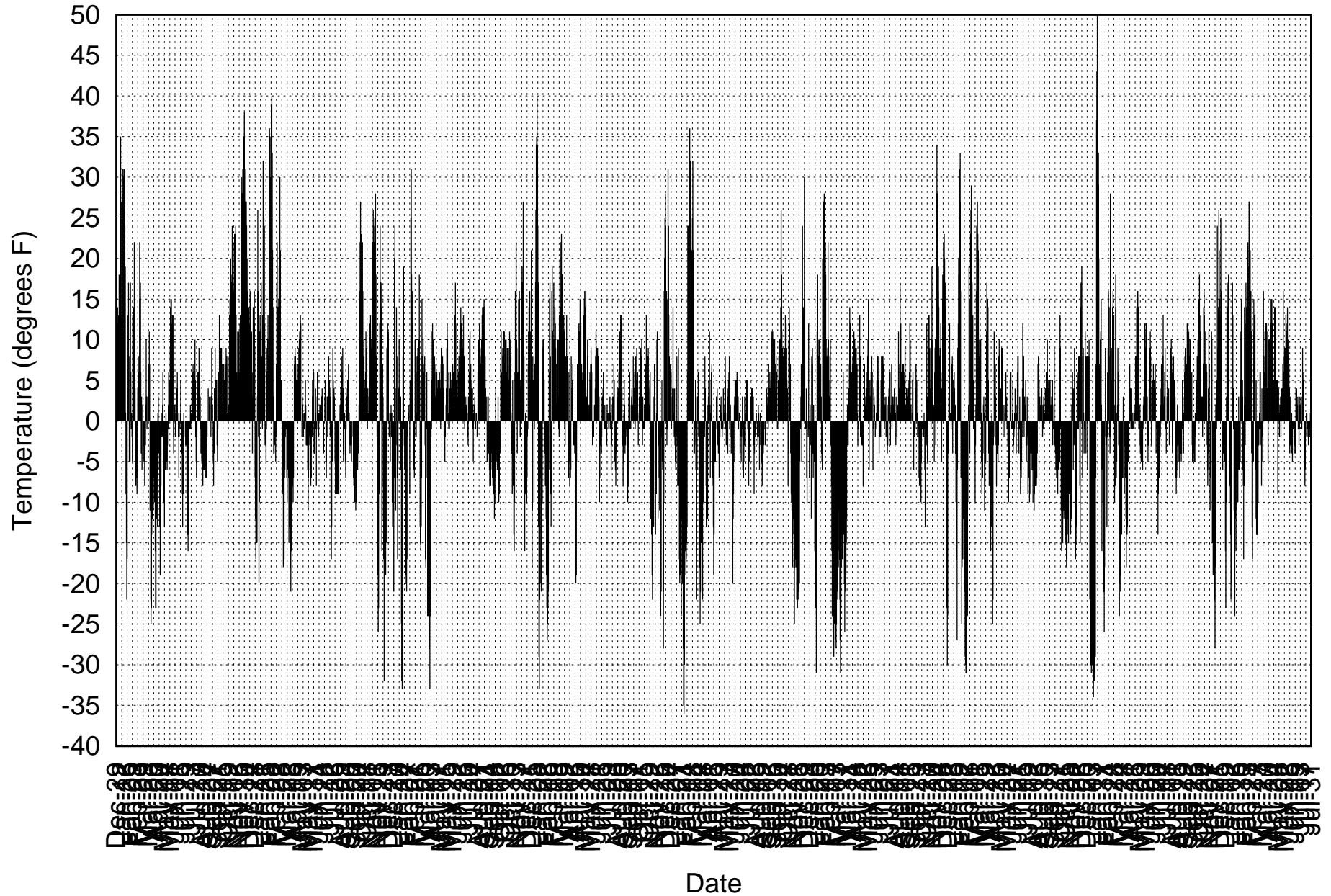
Fairbanks Weather, last 365 days, difference between av daily temp and 31-year av
